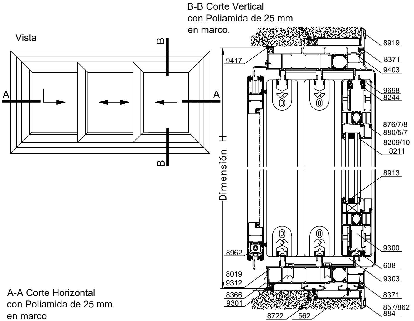
Escala 1:4
