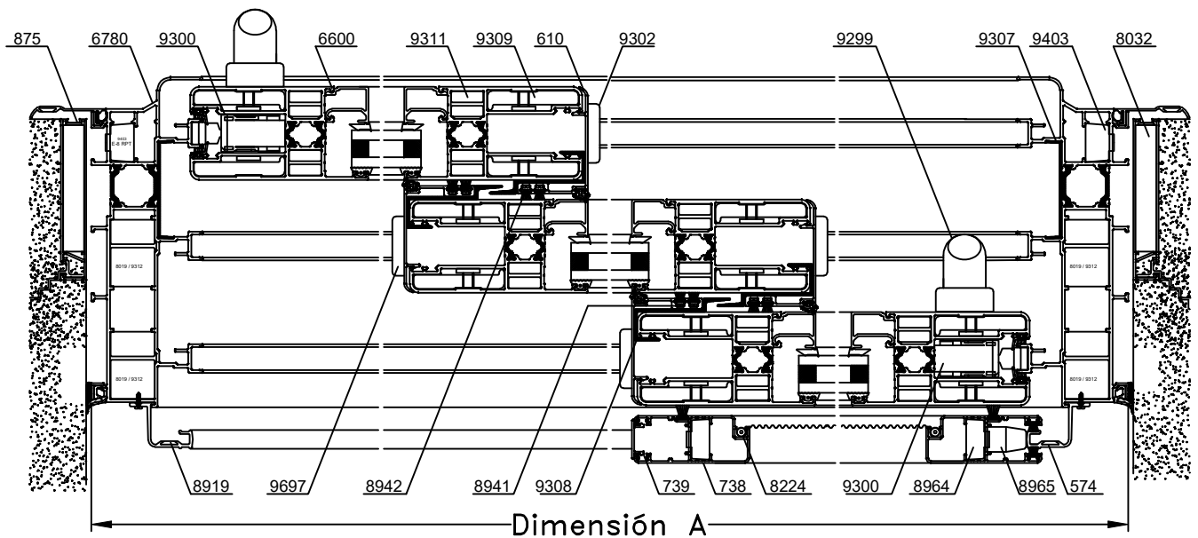
Escala 1:4
